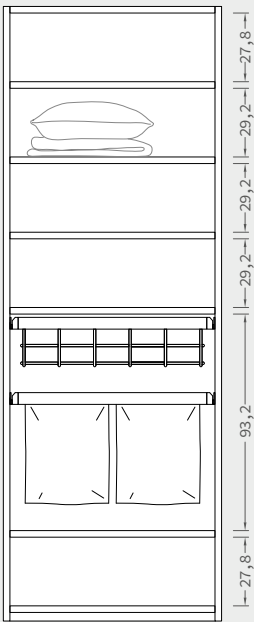
5 ripiani 1 cassetto in filo estraibile 1 coppia cesti estraibili 5 shelves 1 removable drawer 1 couple of removable baskets
