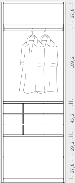
4 ripiani 1 tubo appendiabiti 1 crociera interna 4 shelves 1 coat-hanger 1 inner cruiser
